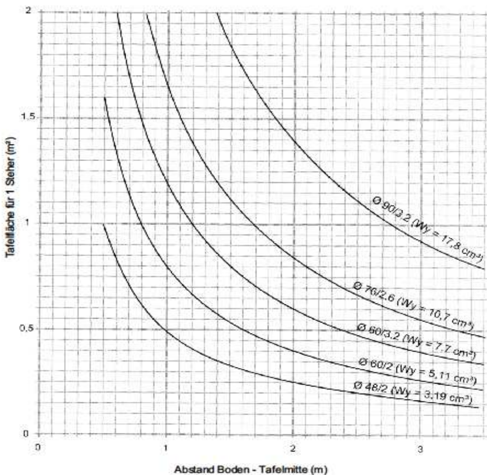
Abbildung 2: Stahlrohre (St 37-2)
