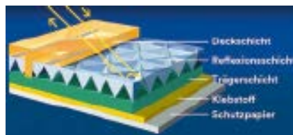
Folie Typ 2 Signalfolie High Intensity Prismatic (HIP) Garantiefrist 10 + 2 Jahre
