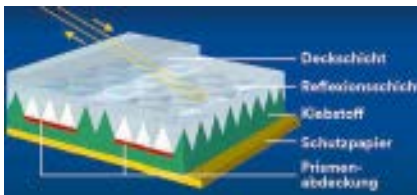
Folie Typ 1 (Digitaldruck) Advanced Engineer Grade Garantiefrist 7 + 2 Jahre
