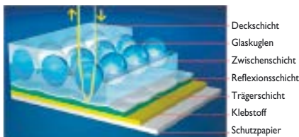
Folie Typ 1 (Siebdruck) Engineer Grade Garantiefrist 7 + 2 Jahre
